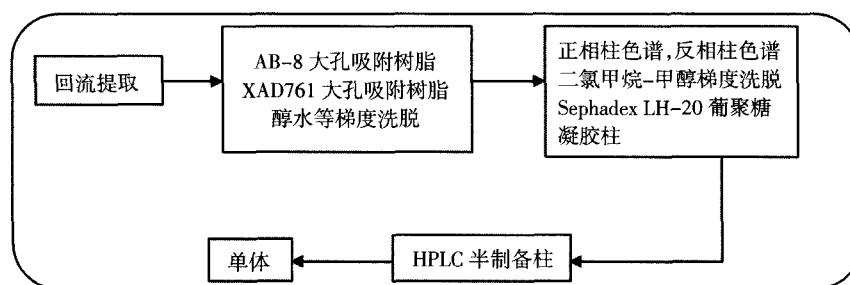
图1 海参皂苷的提取分离流程图
